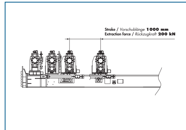
Clamping and breaking devices Klemm- und Brechvorrichtungen
